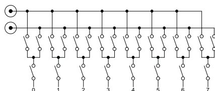
CXE/2x8 Switch Module
